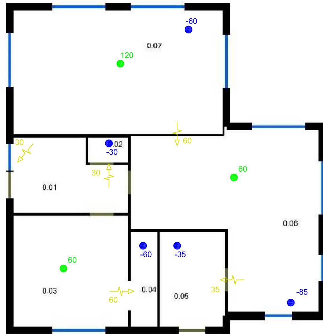
Begane grond
