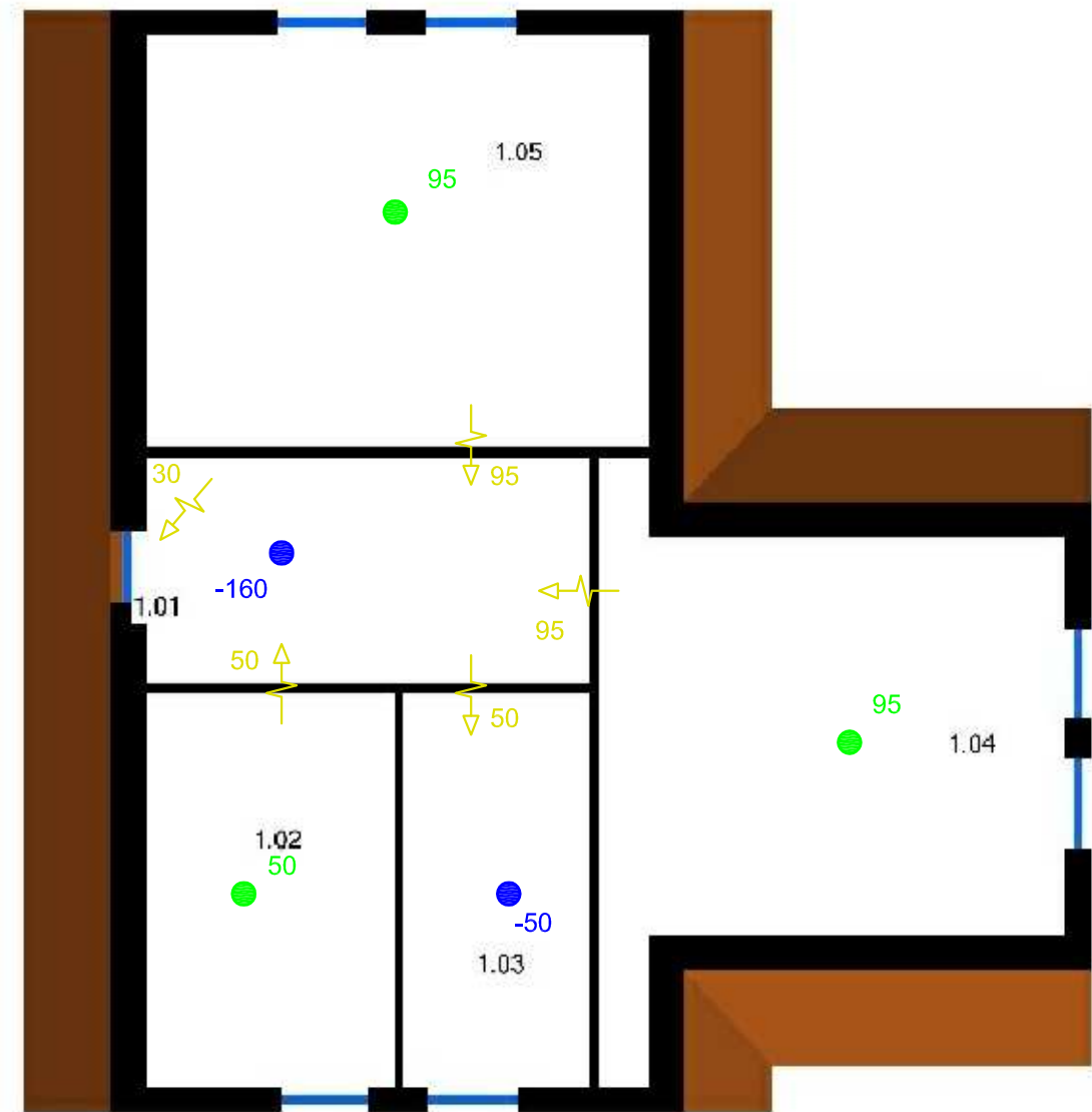
1e verdieping
